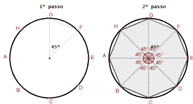
Construção de um octógono regular.
